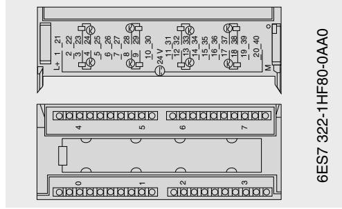
Bild 2/3 Digitalausgabebau- gruppe SM 322-1HF80
