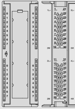
6ES7 322-1BL00-0AA0
