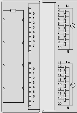
6ES7 322-1EH01-0AA0
