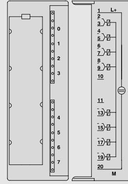
6ES7 322-8BF00-0AB0
