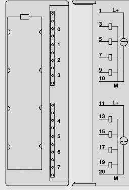
6ES7 322-1BF01-0AA0
