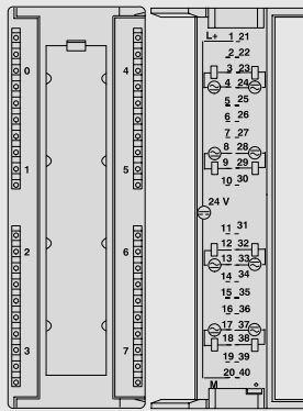
6ES7 322-1HF10-0AA0 6ES7 322-1HF80-0AA0
