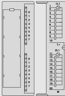
6ES7 322-1HH00-0AA0
