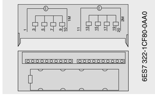
Bild 2/4 Digitalausgabebau- gruppe SM 322-1CF80
