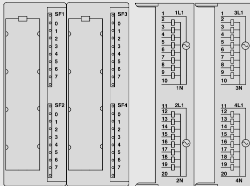
6ES7 322-1EL00-0AA0
